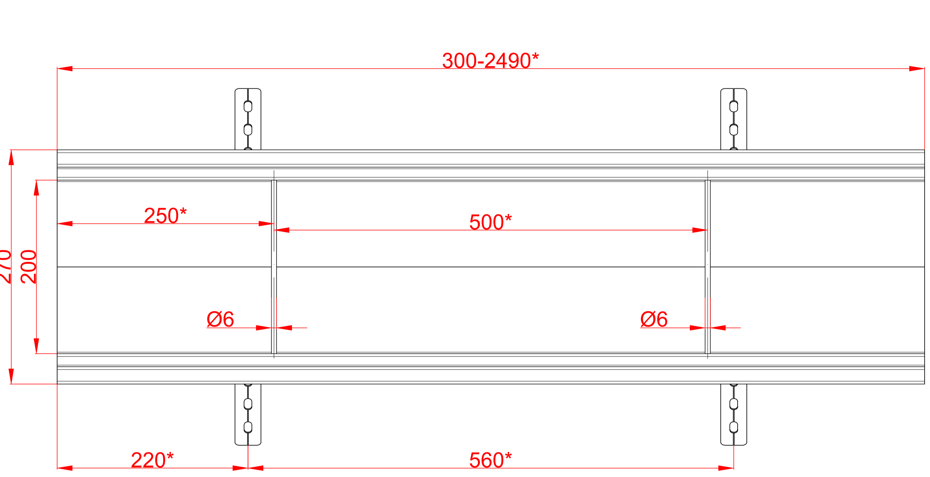
A-A (1:2)
